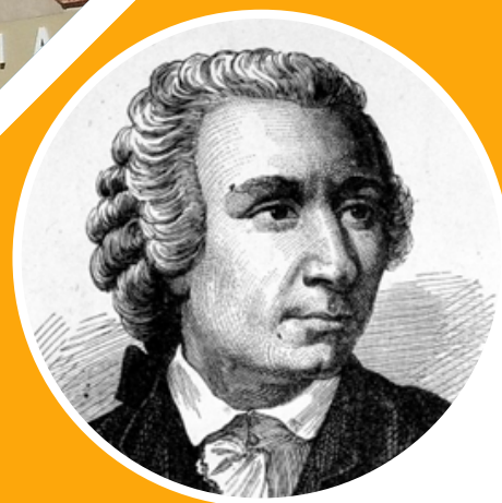
LEONHARD EULER
